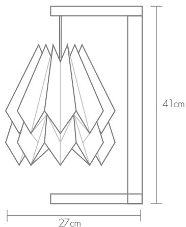
PLAIN TABLE LAMPSHADE CANDEEIRO DE MESA LISO ORI-TA-P-X
